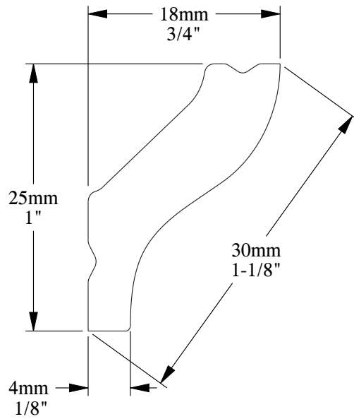
SCALE 2:1
