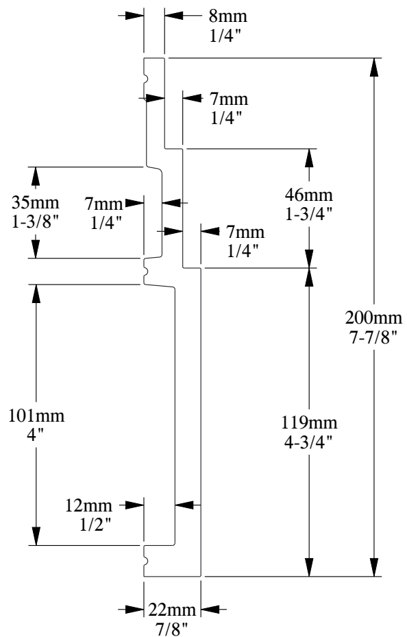
SCALE 1:2
